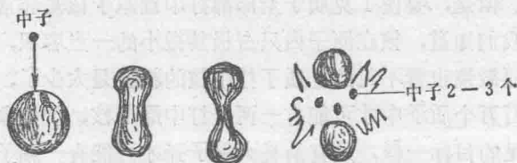
图 1-1 铀-235 核裂变示意图
