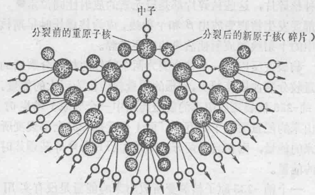
图 1-2 链式反应示意图
