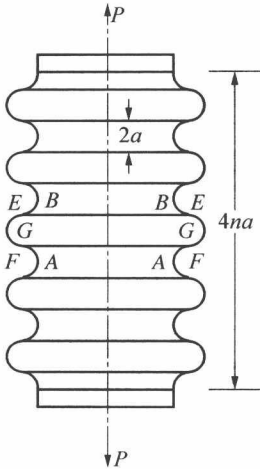
图1 半圆弧波纹管尺寸
