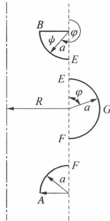
图2 半圆弧波纹管单元坐标
