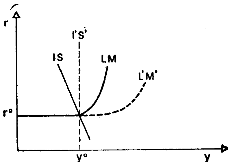
图 3 IS—LM 模型
