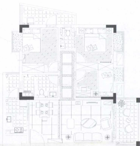
● 平面布置图
