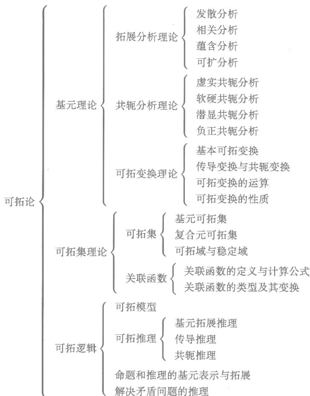
图 1.1 可拓论框架
