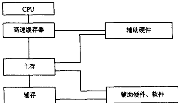
图 1-2 3 级存储器层次结构
