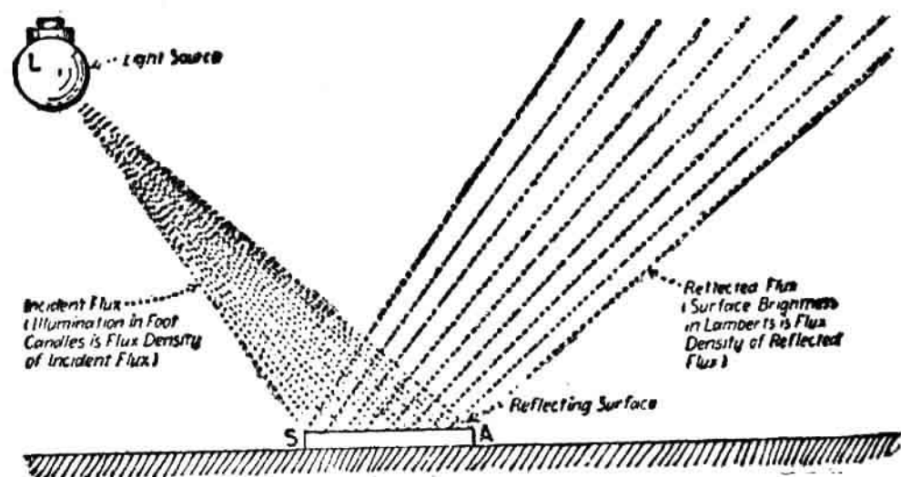
第二圖 平面之反射
