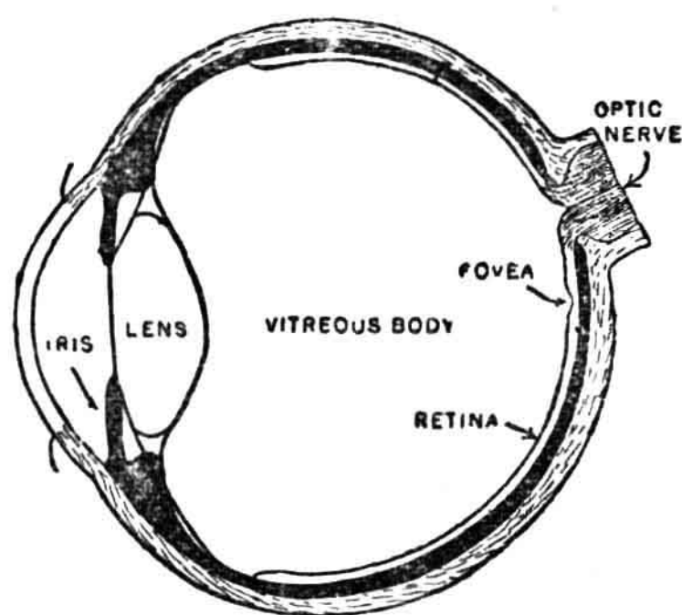
第一圖 眼之剖面
