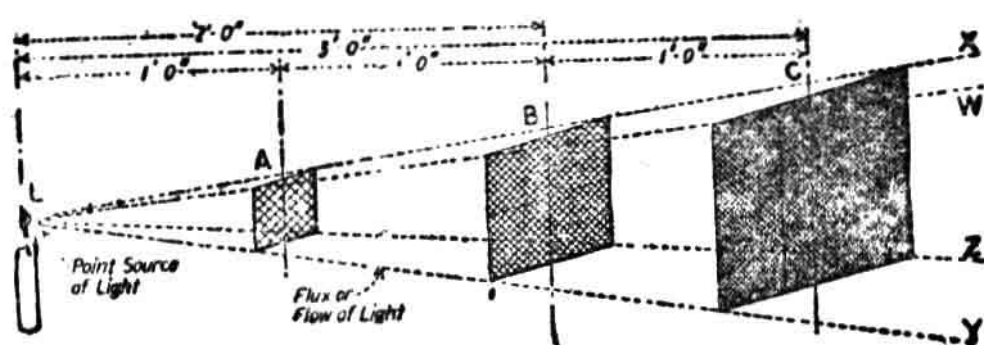
第四圖 光之傳播
