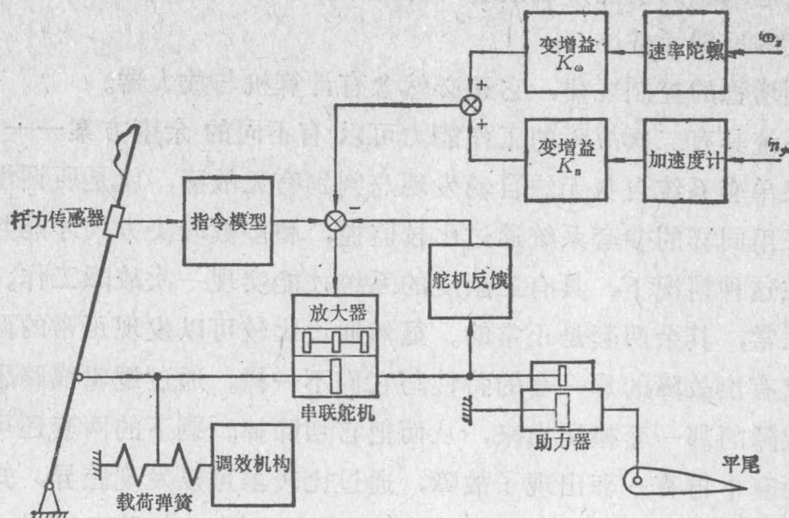
图5-10 典型控制增稳系统联动方块图
