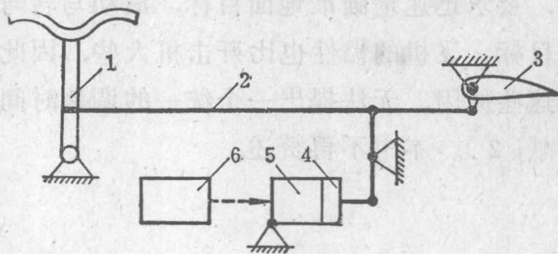
图 5-1 舵机与驾驶杆操纵系统并联
