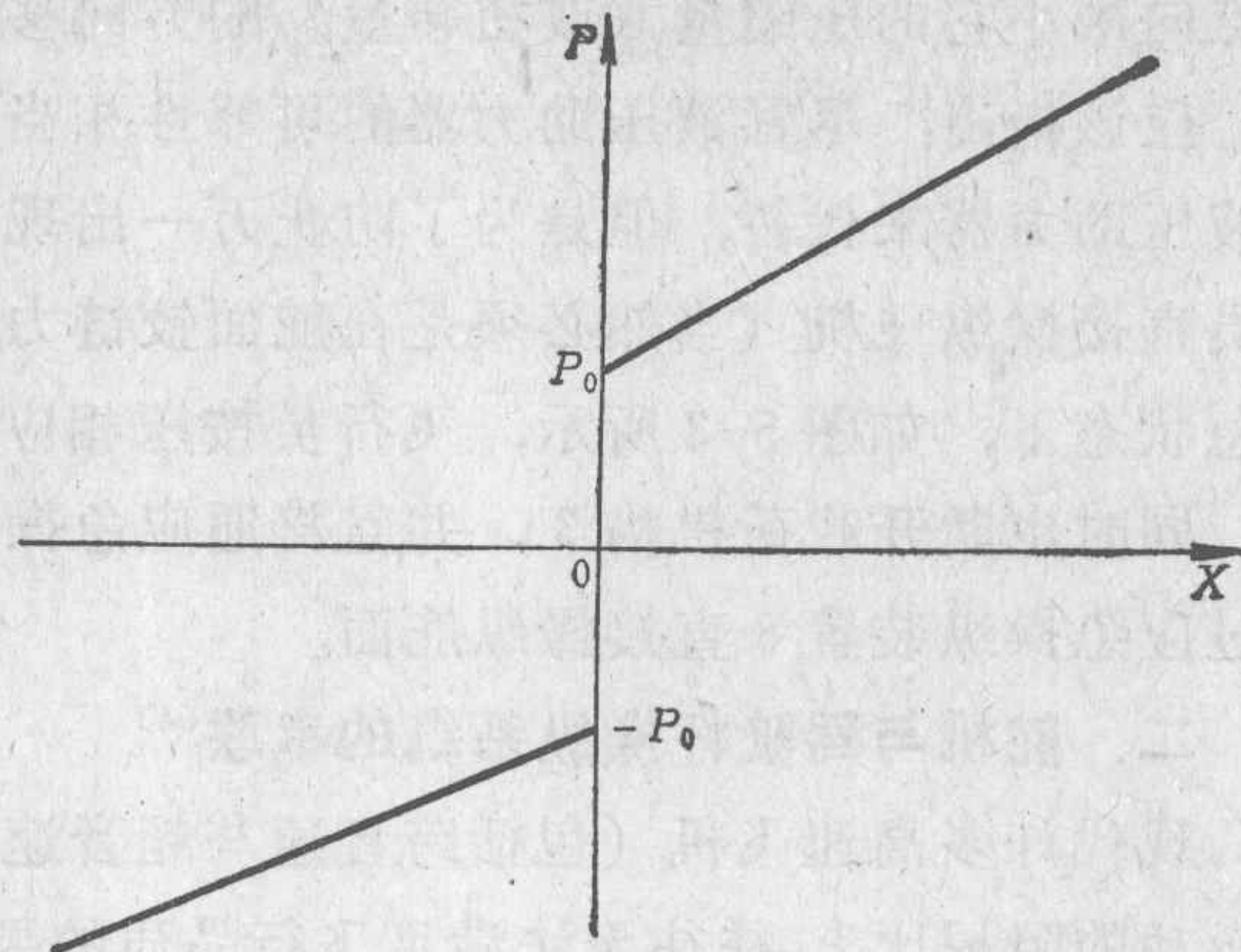
图5-6 具有预载的非线性载荷机构
