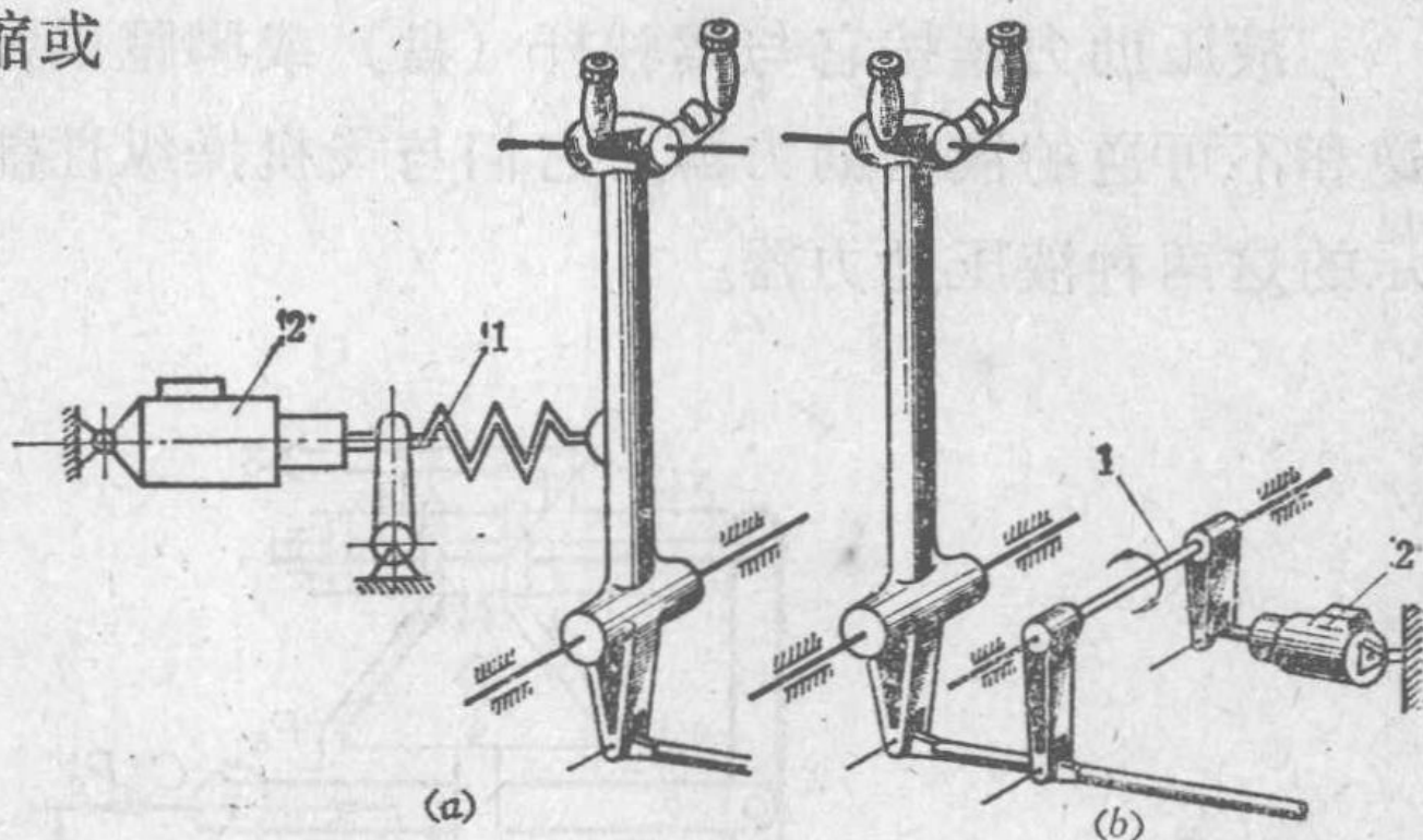
图5-4 调整片效应机构与载荷机构联接示意图
