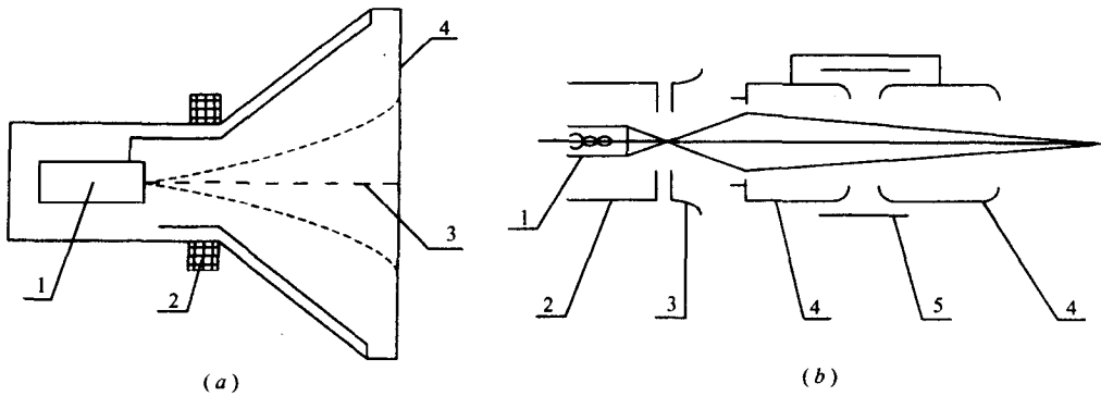
图 1-1 单色显像管的基本结构
