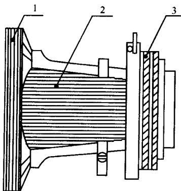
图 1-5 偏转线圈
