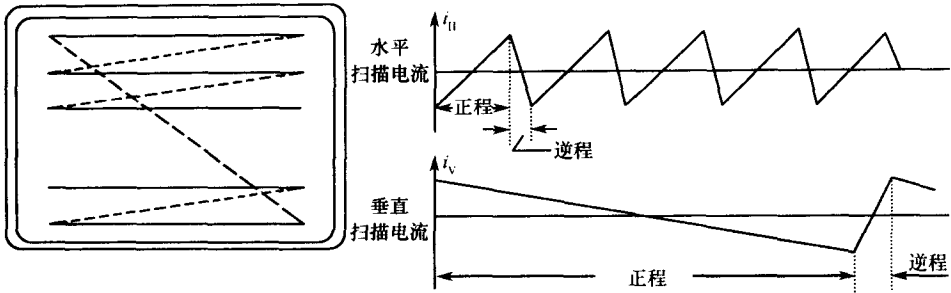
图 1-7 光栅的形成
