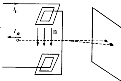
图 1-6 电子束水平偏转的原理
