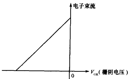
图 1-2 显像管的栅极控制特性
