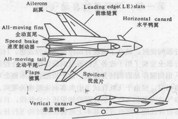
图 0-2 推荐的随控布局飞机
