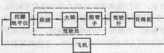
图 0-3 驾驶员控制飞机的方块图
