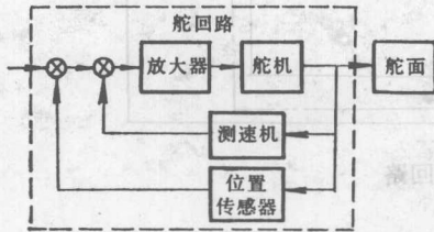
图 0-5 舵回路
