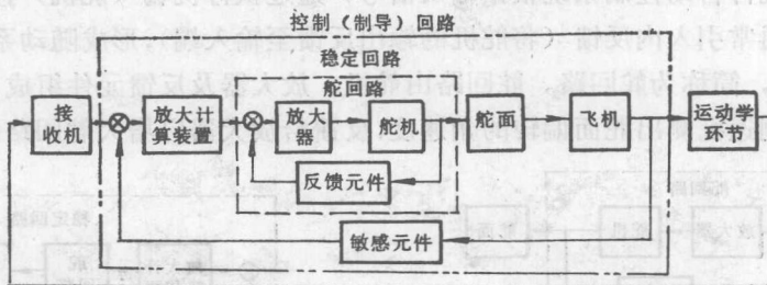
图 0-8 控制(制导)回路
