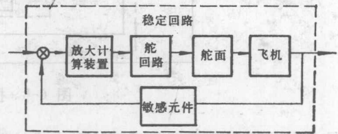
图 0-6 稳定回路
