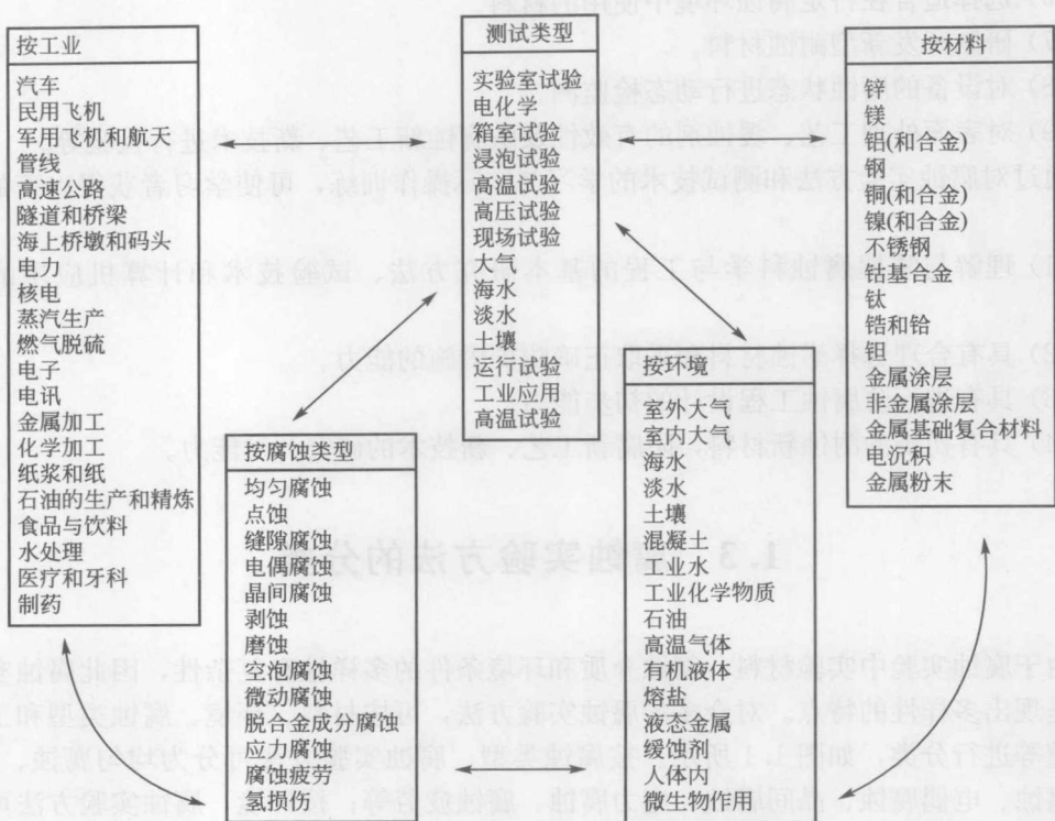
图 1.1 腐蚀实验方法的分类
