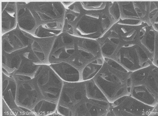
图 1.2 三维网状泡沫体形貌示例
