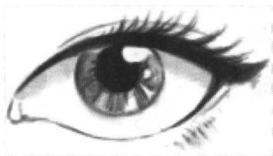
图 1-13 擦掉虚线
