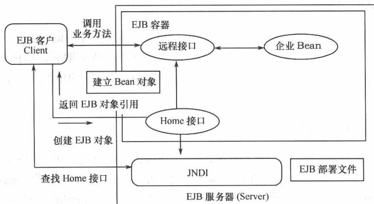
图 1.4 EJB 的调用过程
