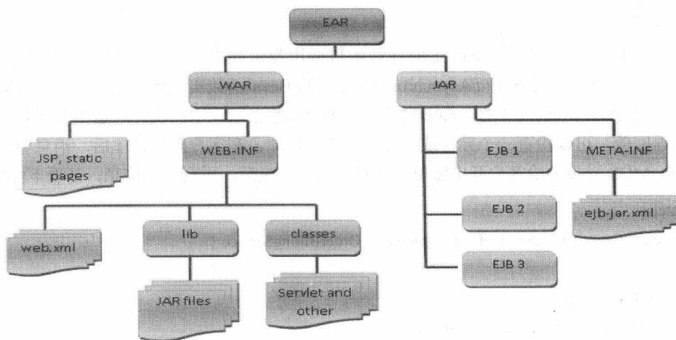
图 1.1 EJB 3.0 打包方式结构图
