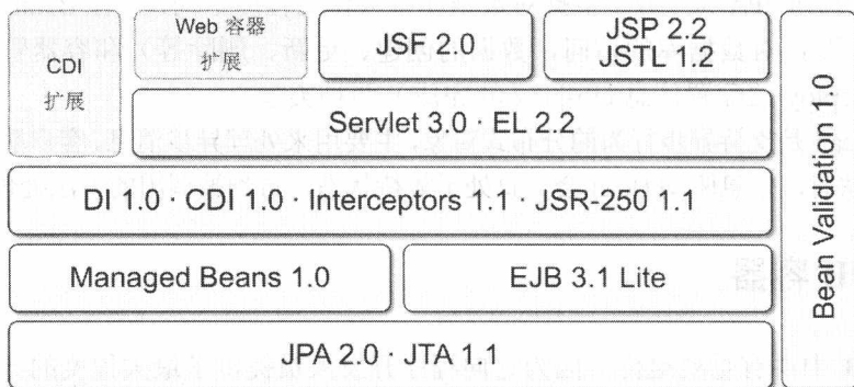
图 1.3 EJB 3.1 在 Java EE 6 体系结构中的位置
