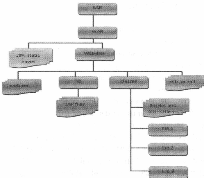
图 1.2 EJB 3.1 的打包方式结构图
