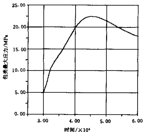
图 8 包壳最大应力随时间变化的特性曲线 (失水事故工况)
