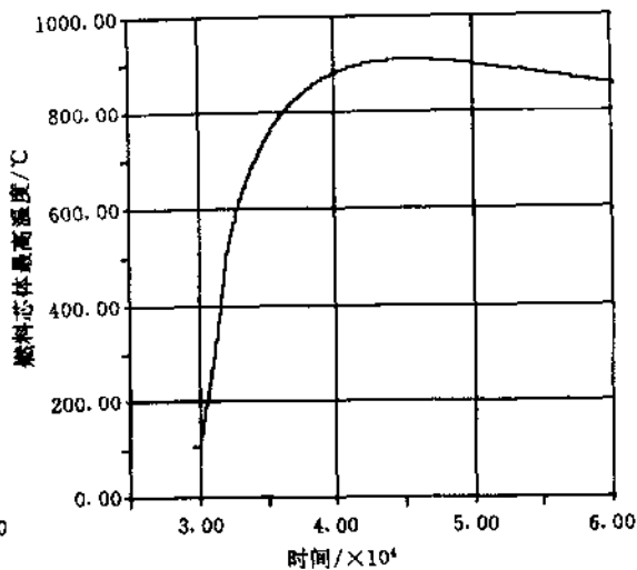
图7 燃料芯体最高温度的瞬态特性曲线 (失水事故工况)
