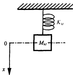
图 1-1 质量—弹簧系统
