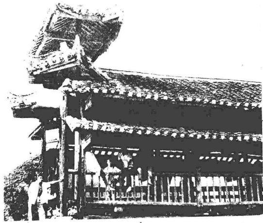
新业乡芙蓉坝土家族风雨桥
