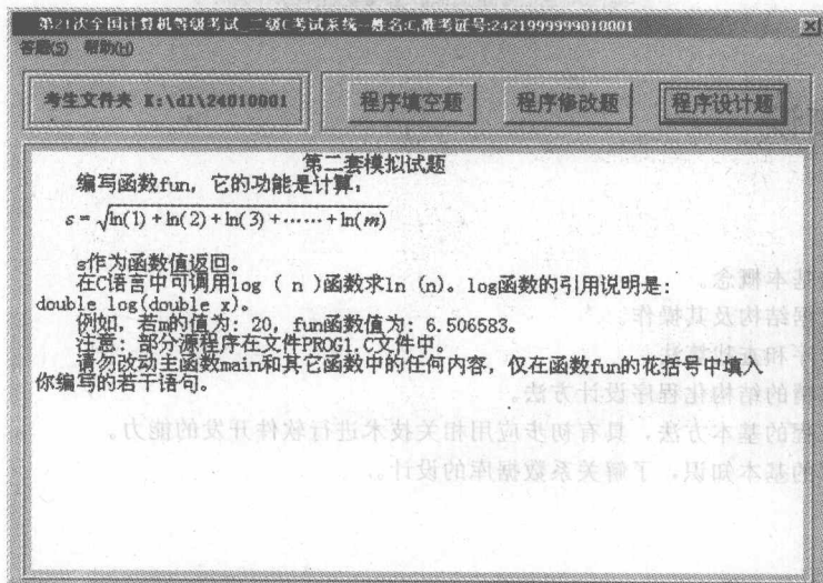
图 0-11 程序设计题
