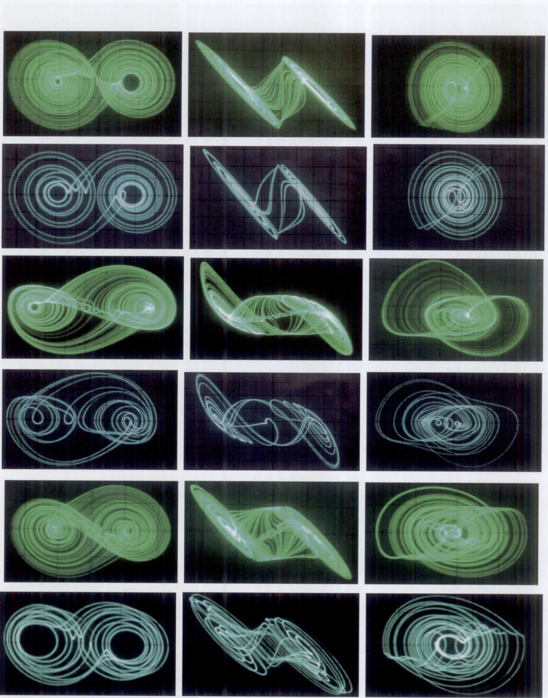
彩图6 三阶级联反相积分器电路相图,前2行为阶跃非线性,中2行为三次方非线性,后2行为标准限幅非线性。 每2行中第1行时间常数为0.1 ms,第2行时间常数为1 ms;由左向右依次为 x-y 相图、 x-z 相图、 z-y 相图
