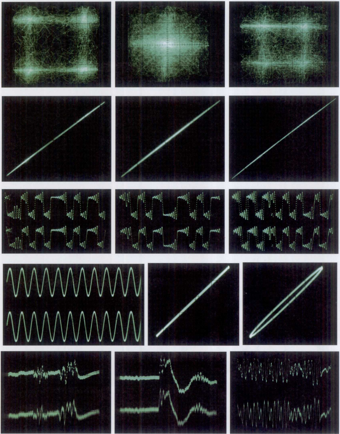
彩图9 混沌保密通信电路示波器显示图。第1行为不同步相图,第2行为同步相图(由左向右依次为 x_1-x_2 、 y_1-y_2 、 z_1-z_2 相图),第3行为 x_1-x_2 同步波形图,第4行为调制与解调信号,第5行为发送端输入调制信号和接收端解调输出信号
