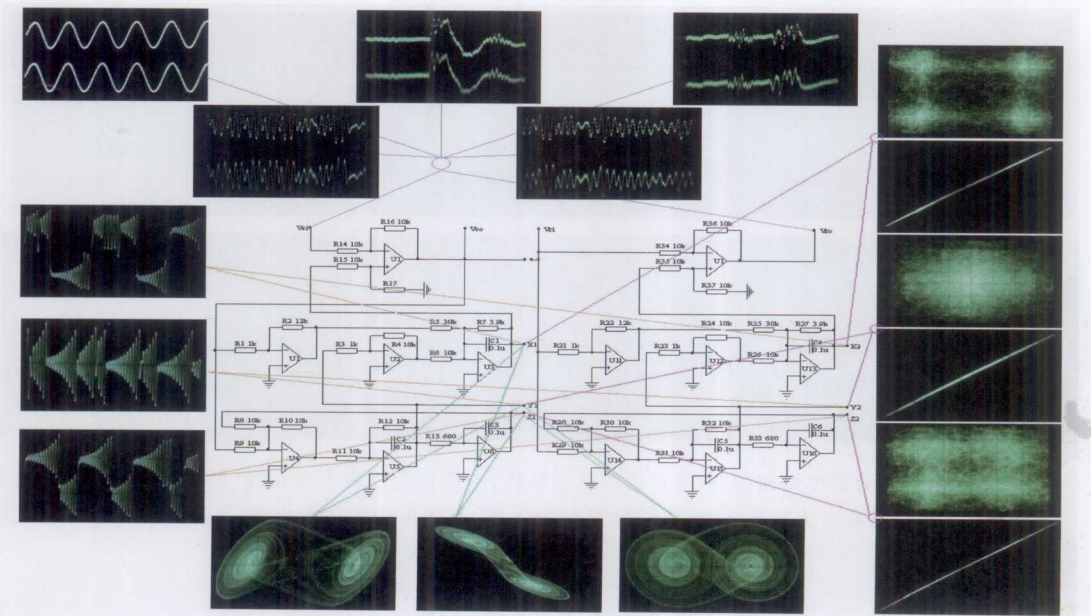
彩图 8 混沌保密通信电路与示波器显示的位置波形
