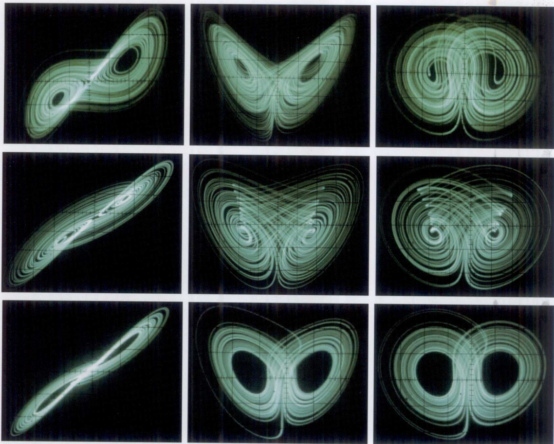
彩图4 洛伦兹(上)、陈关荣(中)、吕金虎(下)方程电路相图(由左向右依次为 x-y 、 x-z 、 z-y 相图)
