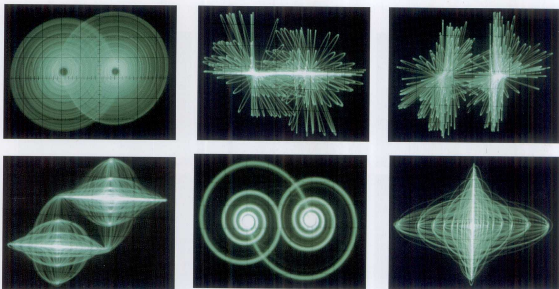
彩图5 限幅非线性混沌电路输出的相图(由左上至右下依次为 x_2-x_1 、 x_2-x_4 、 x_3-x_1 、 x_3-x_2 、 x_3-x_4 、 x_4-x_1 相图)
