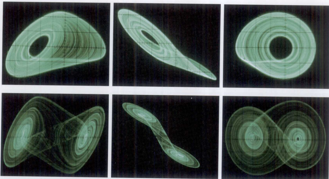
彩图 1 蔡氏电路单涡漩(上)与双涡漩(下)混沌相图(由左向右依次为 x-y 相图、 x-z 相图、 z-y 相图)
