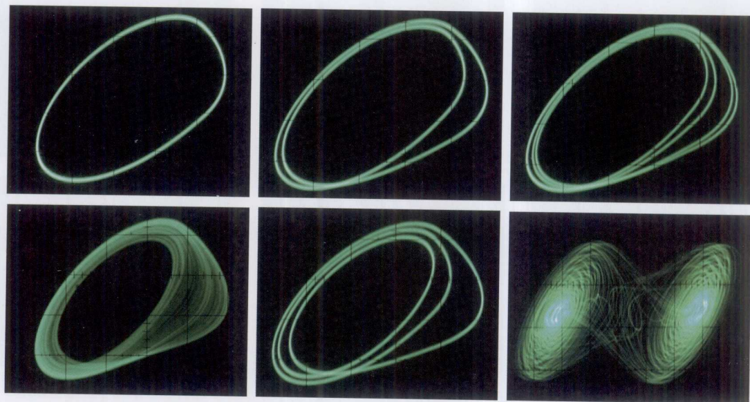
彩图 3 基本蔡氏电路混沌演变图(周期 1、周期 2、周期 4、单涡漩、周期 3、双涡漩)
