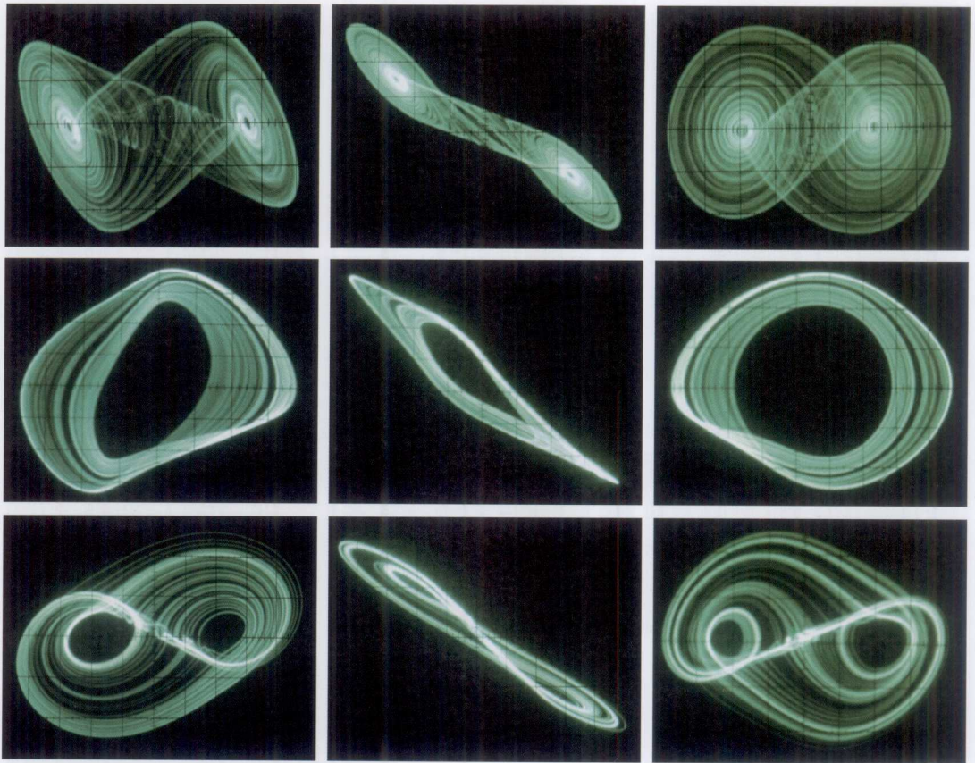
彩图 7 三种 CNN 电路混沌电路输出的相图(由左向右依次为 x_1-x_2 、 x_1-x_3 、 x_2-x_3 相图)
