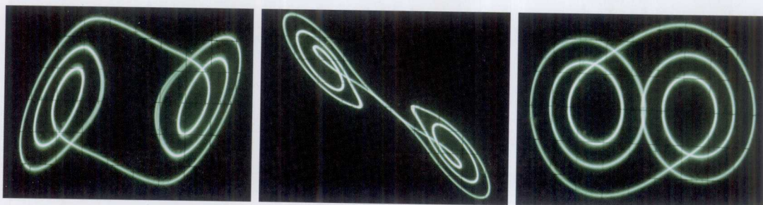
彩图 2 蔡氏电路双涡漩中的周期窗口相图(由左向右依次为 x-y 相图、 x-z 相图、 z-y 相图)
