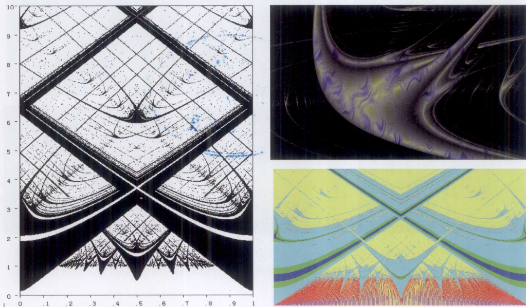
彩图 12 圆周映射分岔图
