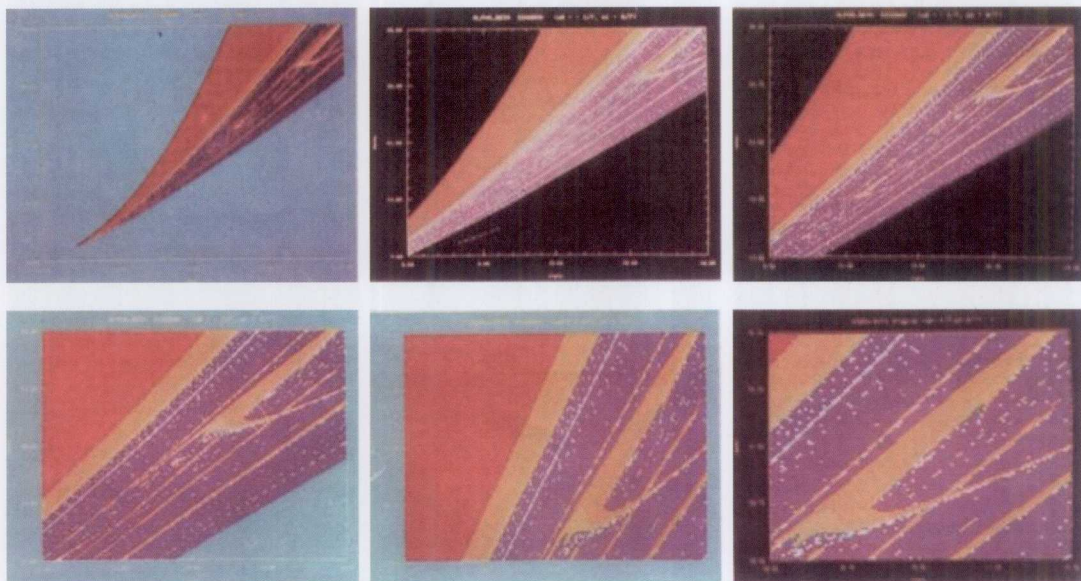
彩图 11 蔡氏电路 \alpha - \beta 平面分岔的逐级放大图 [36]
