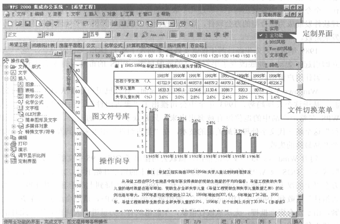
图 1.2.1 WPS 2000 首创的编辑方式
