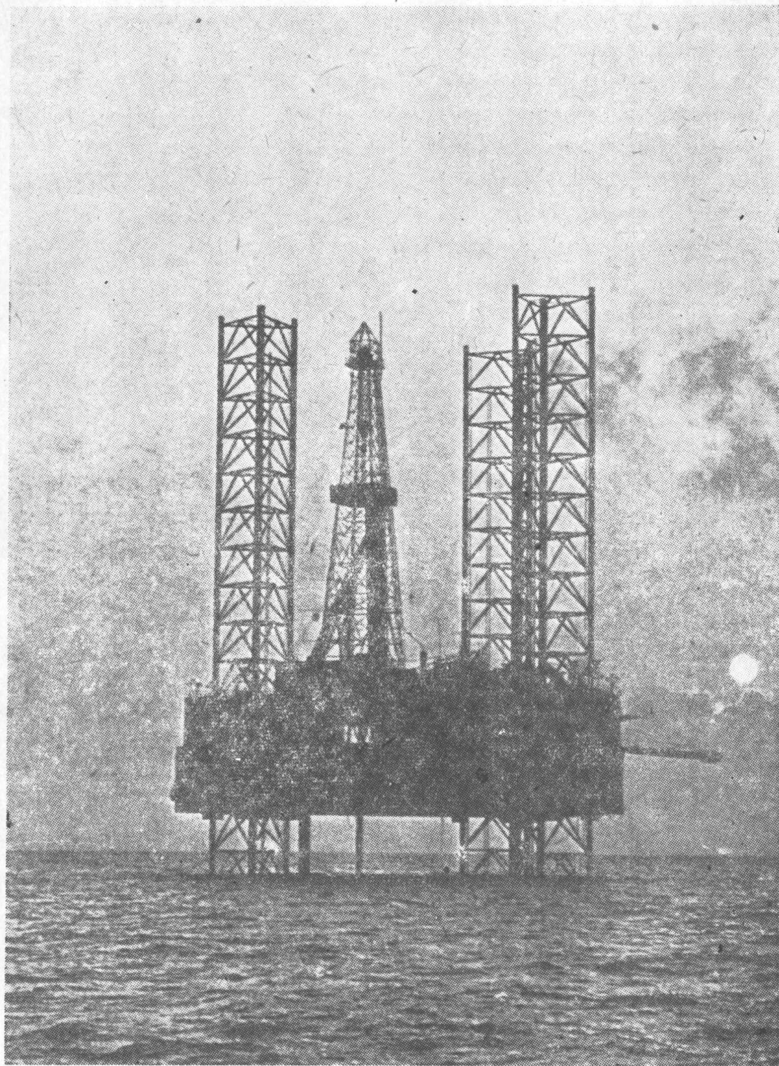
北部湾海上钻井平台
