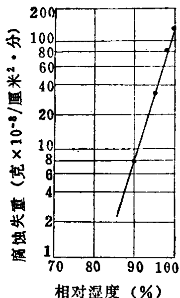
图1 钢铁腐蚀失重与相对湿度的关系
