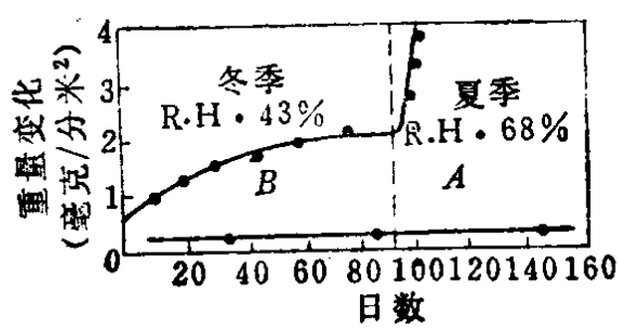
图 3 钢铁在大气中的腐蚀
