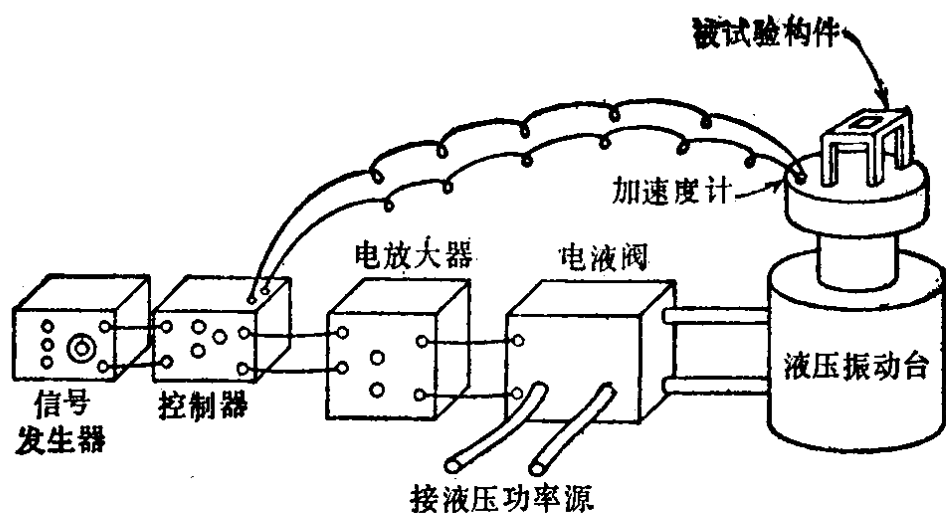
图1.2 振动试验系统
