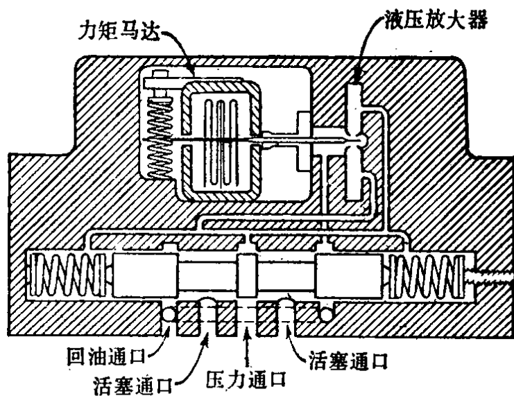
图1.3 电液阀
