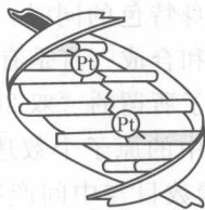
图2 配合物与DNA作用示意图
