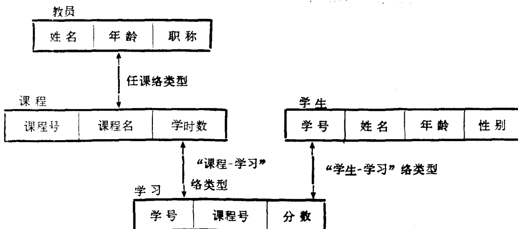
图1.4 数据的网络模型
