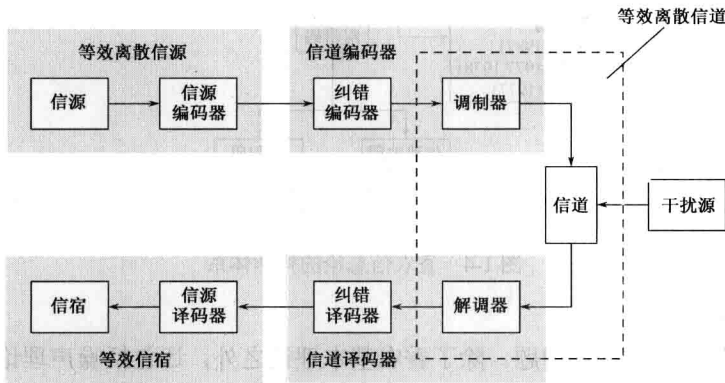
图 1-3 通信系统模型的细分
