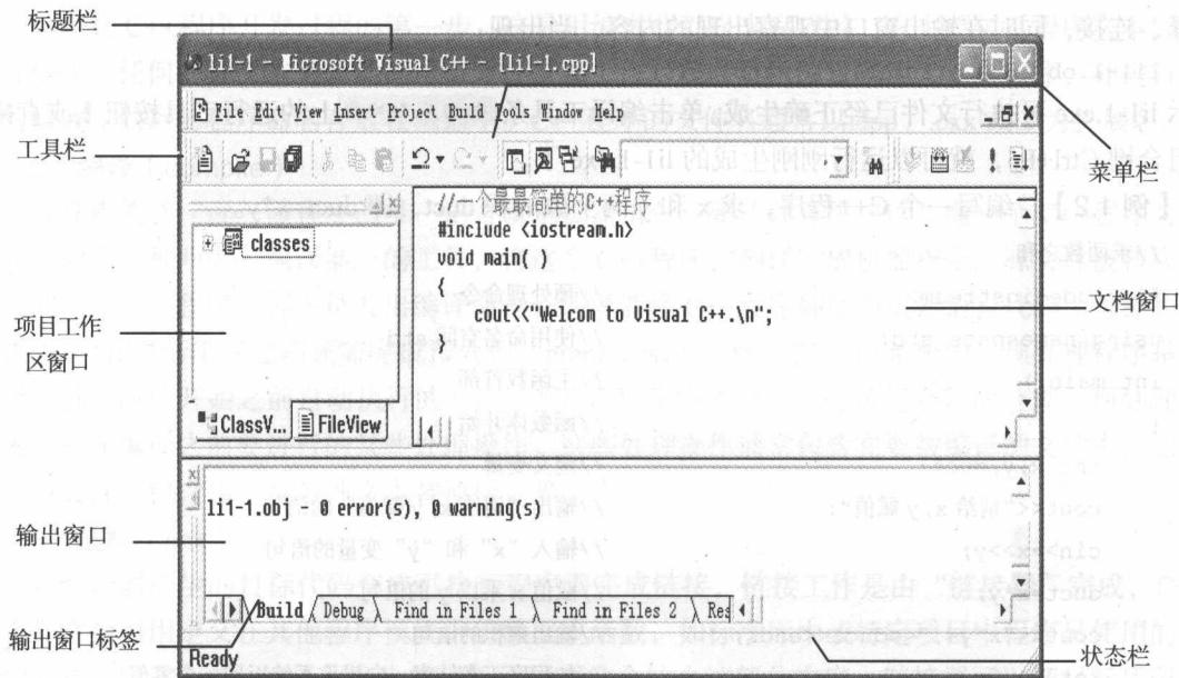
图 1.3 Visual C++ 6.0 开发环境
