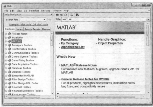
图 1.1.3 帮助主窗口
