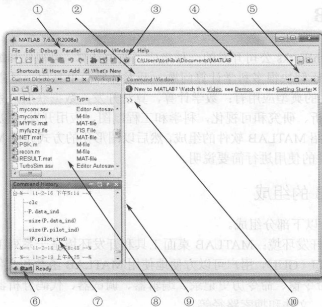
图 1.1.1 MATLAB 主界面
