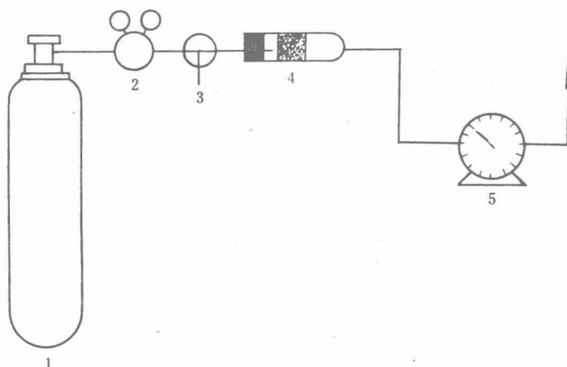
图2 测定装置
