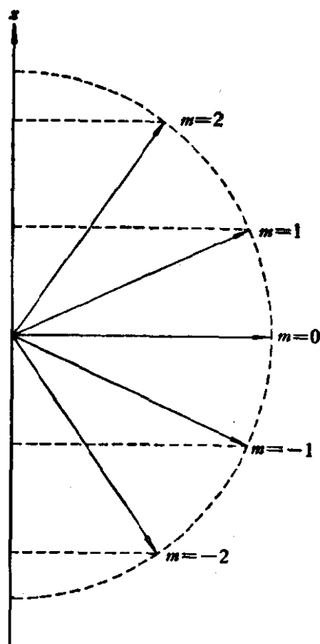
图 1-1 核磁的取向(以 I=2 为例)
