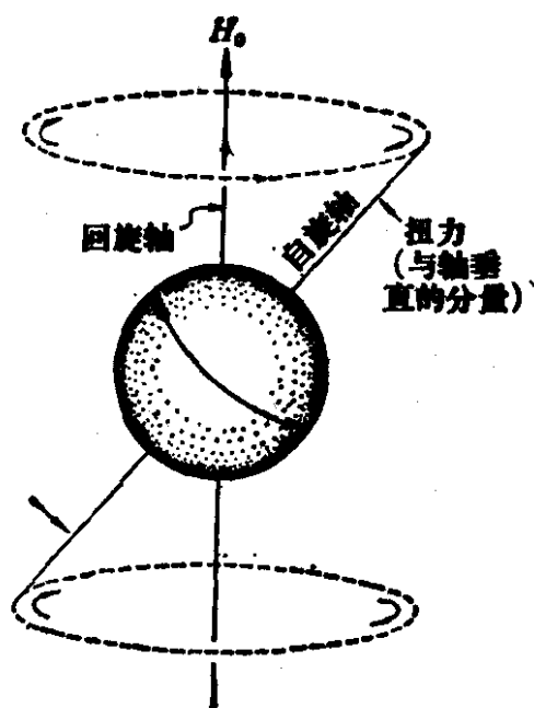
图 1-2 原子核的自旋
