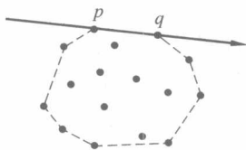
图 1-6 相对于 \text{CH}(P) 边界上任一边所在的直线, P 中所有点均居于同侧
