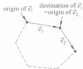
图 1-7 确定 E 中各边的次序
