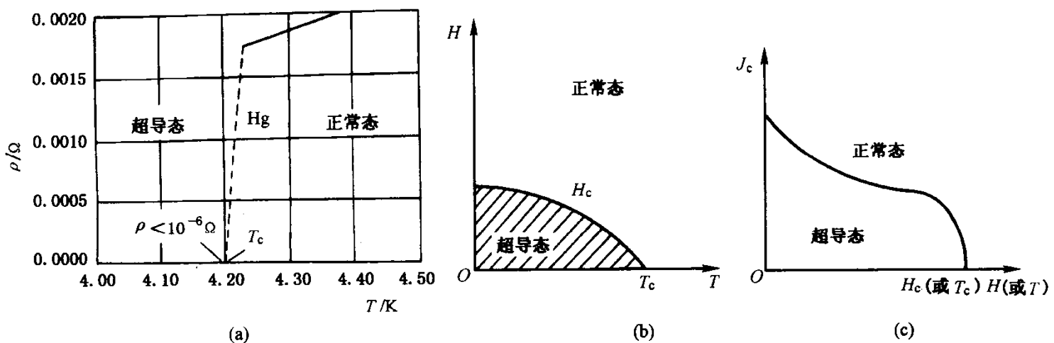
图 1-2 \rho 、 H 、 J 与温度关系示意图
