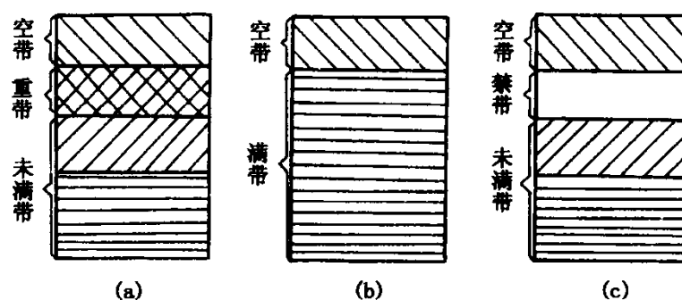
图 1-1 导体的能带结构
