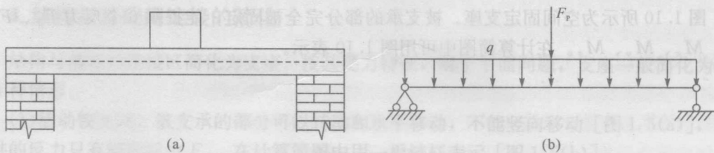
图 1.11 简支梁计算简图
