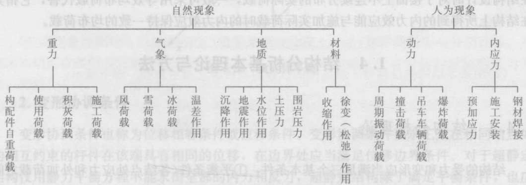
图 1.25 结构荷载
