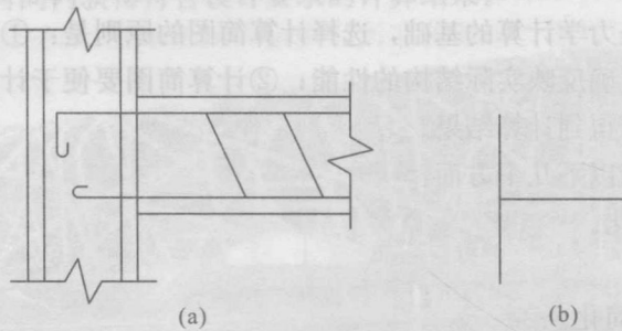
图 1.4 刚结点
