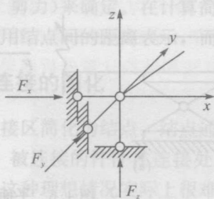
图 1.9 空间固定铰支座
