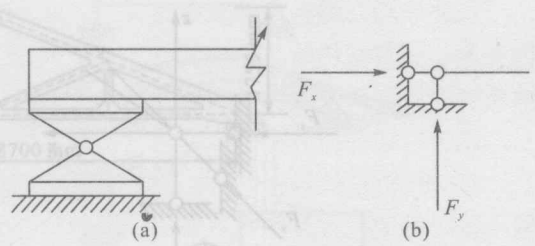
图 1.6 平面固定铰支座
