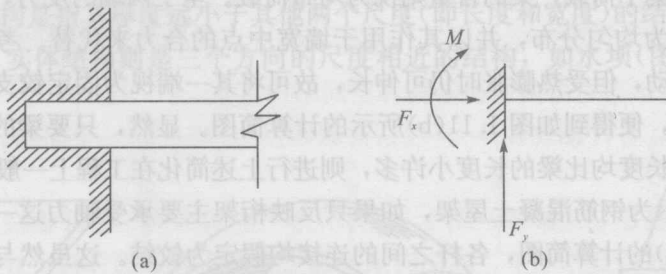
图 1.8 平面固定支座
