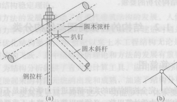
图 1.3 铰结点
