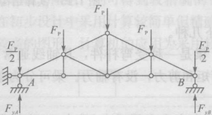
图 1.22 平面桁架
