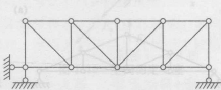
图 1.19 桁架
