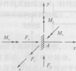
图 1.10 空间固定支座
