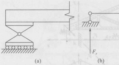
图 1.5 平面活动铰支座
