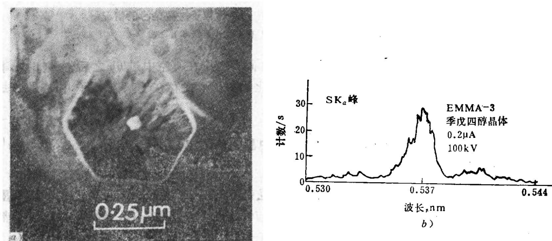
图1-7 修珀希德孕育试样萃取基体粒子的EMMA-3仪分析结果
