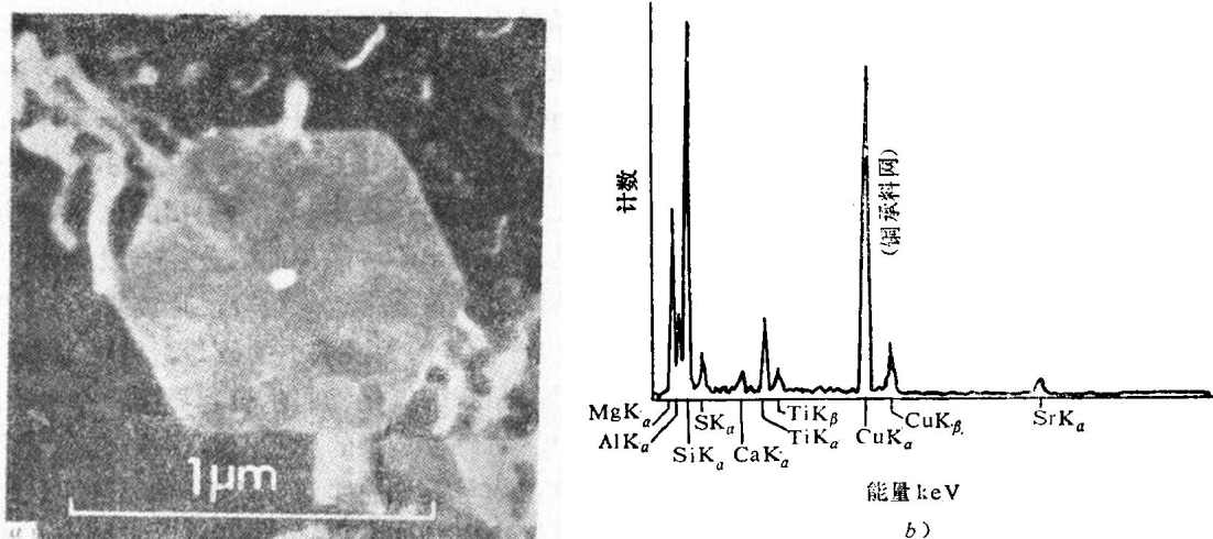
图1-8 富铈修珀希德孕育试样萃取基体粒子的EMMA-3仪分析结果 a) 暗场显微照片, 由发生于中心硫化物核心的反射光摄得 b) 中心区域的能量分散X射线谱
