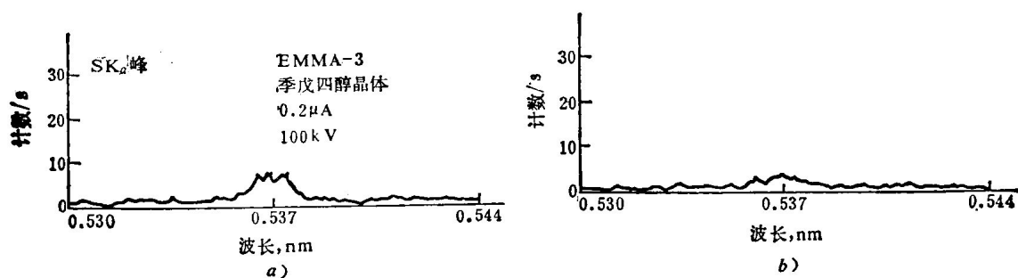
图1-6 萃取于铸造级孕育的铸铁试样中的基体粒子被硫染污的情况
