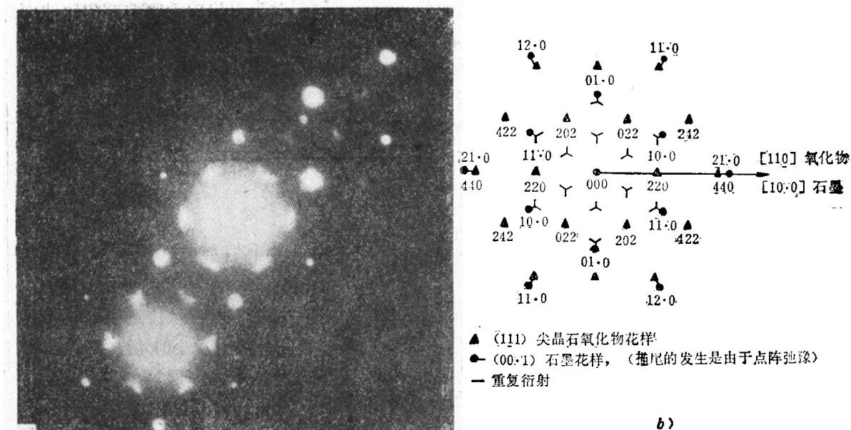
图1-5 图1-4 a 所示的基体粒子的电子衍射分析
