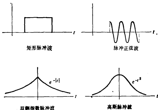
图 1.2 几种能量信号
