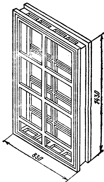
图 1.6 放置底板的框架
