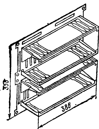
图 1.5 安装典型可更换逻辑元件的底板
