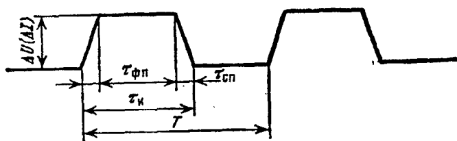
图 1.2 离散（脉冲）信号
