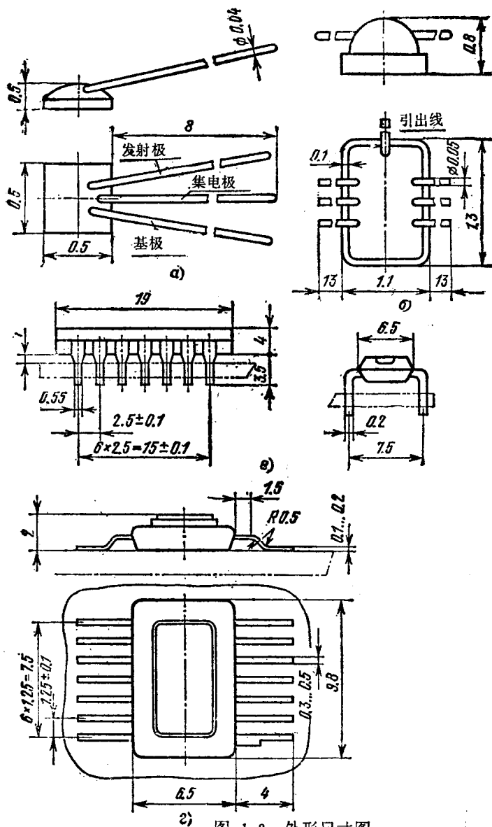
图 1.3 外形尺寸图
