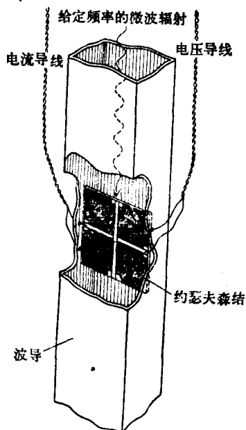
图1 用已知频率的微波激发约瑟夫森结,测定 e/h 值。约瑟夫森结放在装有液氮的杜瓦瓶内的波导里。微波感生电流在电流-电压图上形成阶梯,这是约瑟夫森结的特征(见右图)。通过电流导线加一“偏压”到结的这些阶梯之一上,办法是用可调节的电流源(用几个可变电阻与一个电池组),通过电压导线加上去的。阶梯的电压可用电位计测定。微波频率与此阶梯电压成正比,比率就是 2e/h 。
