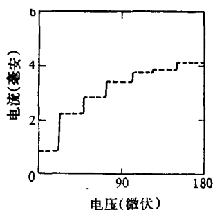
图1 用已知频率的微波激发约瑟夫森结,测定 e/h 值。约瑟夫森结放在装有液氮的杜瓦瓶内的波导里。微波感生电流在电流-电压图上形成阶梯,这是约瑟夫森结的特征(见右图)。通过电流导线加一“偏压”到结的这些阶梯之一上,办法是用可调节的电流源(用几个可变电阻与一个电池组),通过电压导线加上去的。阶梯的电压可用电位计测定。微波频率与此阶梯电压成正比,比率就是 2e/h 。
