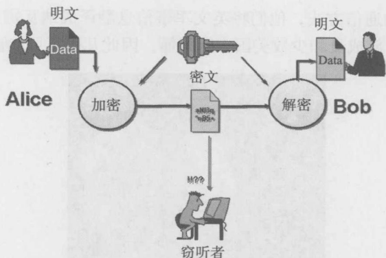
图 1.2 密码学
