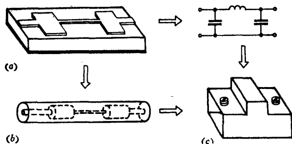
图 1.1 传输线构成的微波电路元件
