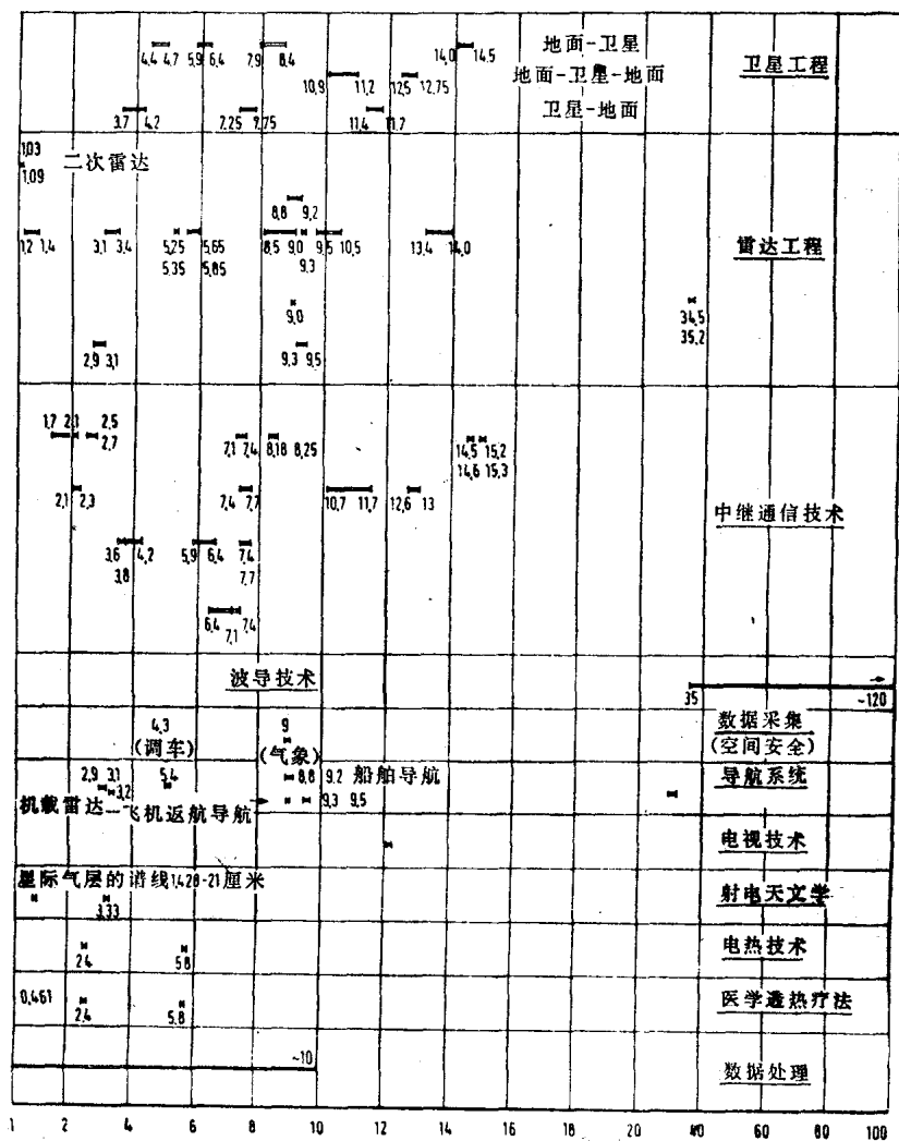
图 1.2 微波技术的各个频率范围
