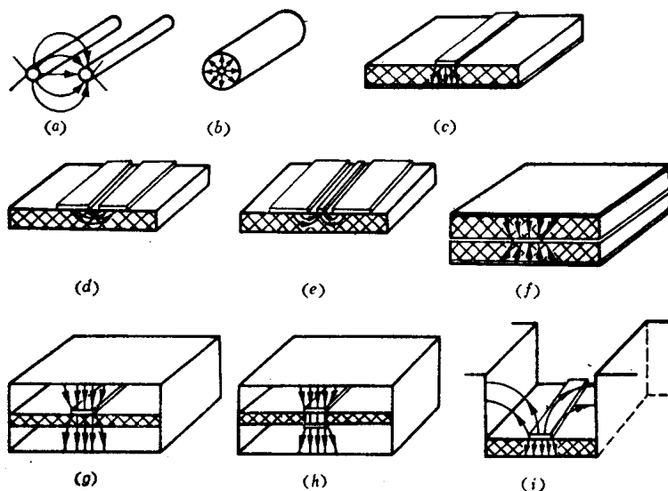
图1.3 TEM 传输线
