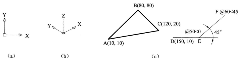
图 1.10 世界坐标系及坐标值的确定
