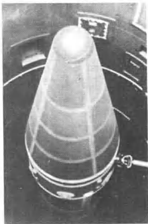
位于发射井中的法国 S—3 陆基战略弹道导弹。该导弹射程 3000 公里,最大发射重量 25.9 吨,核弹头为 120 万吨梯恩梯当量。
