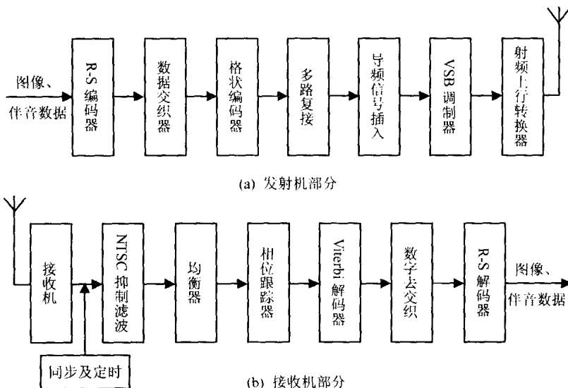
图 1.1.8 VSB 调制数字电视传输系统
