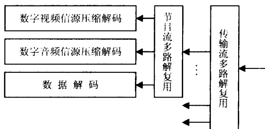
图 1.1.3 信宿部分组成
