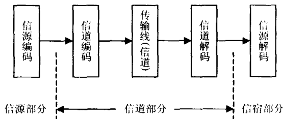
图 1.1.1 数字通信系统组成
