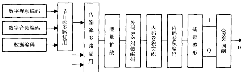
图 1.1.5 数字电视卫星传输系统
