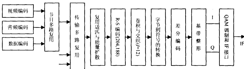
图 1.1.6 数字电视有线传输系统
