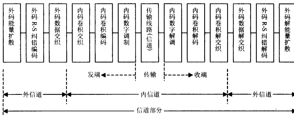
图 1.1.4 信道部分详图
