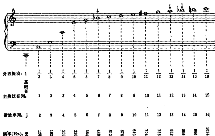
图 1-7 建立在c音上的复合乐音
