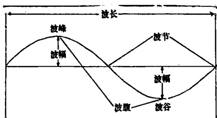
图 1-2 波峰、波谷、波幅、波腹、波长示意
