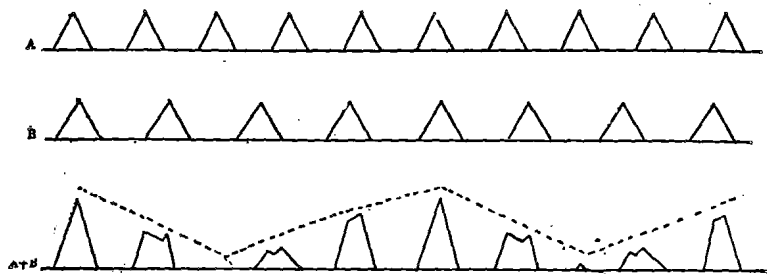
图 1—4 图中虚线表示拍音出现的情况
