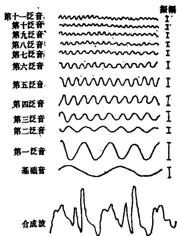
图1—8 乐音分析
