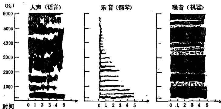
图 1—6 人声、乐音、噪音声谱对比
