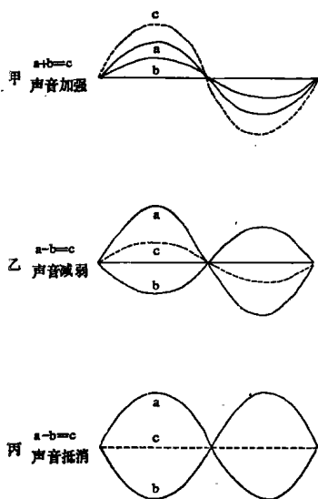
图1-3 波的迭加
