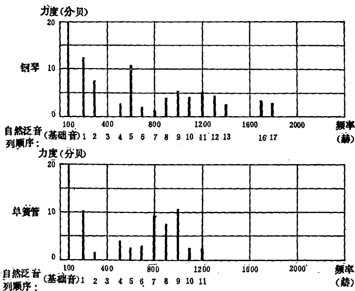
图 1—9 钢琴与单簧管音色分析比较
