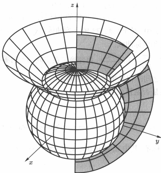
图 2 球面坐标系, a_1 = a_2 = a_3 = 1
