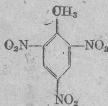
2,4,6-三硝基甲苯
