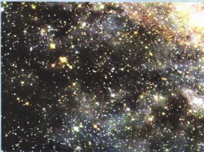
● 美国天文学家哈勃曾把附近的星系分为三种基本结构类型:椭圆星系、旋涡星系和不规则星系
