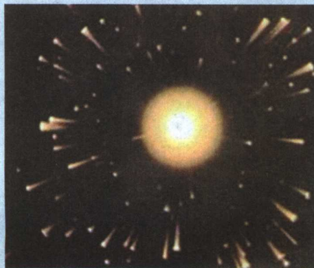
● 大爆炸时的宇宙
