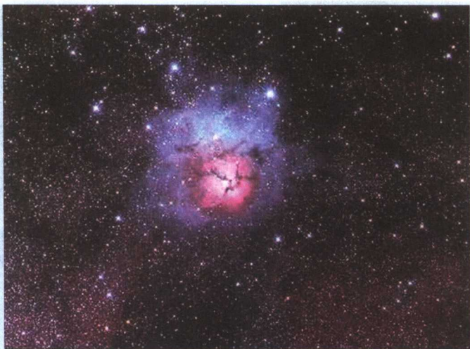
● 弥漫在太空中的星云
