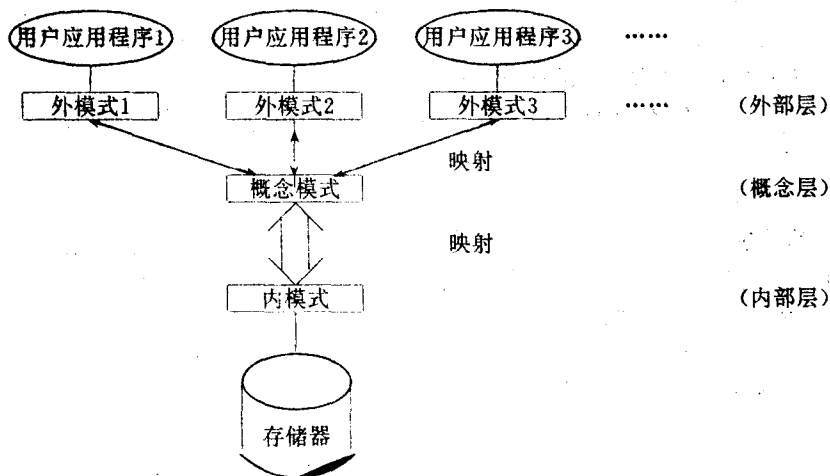
图 1.1 层次体系
