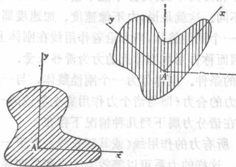
图 6.1-1 刚体的平面平行运动可看作其上任一点 A 的平面运动与绕过 A 点轴线的定轴转动的组合
