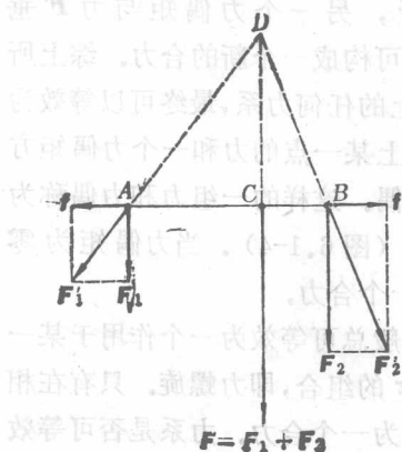
图 6.1-2 求平行力的合力
