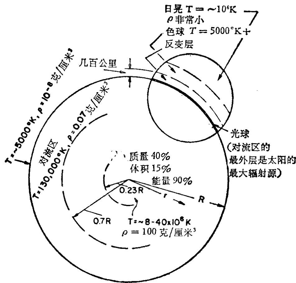
图 1.1.1 太阳结构示意图
