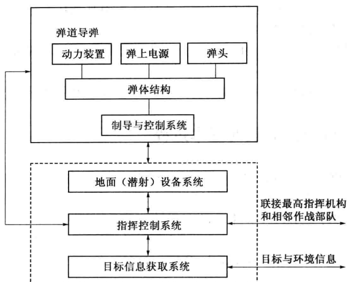
图 1-1 弹道导弹武器系统基本组成图
