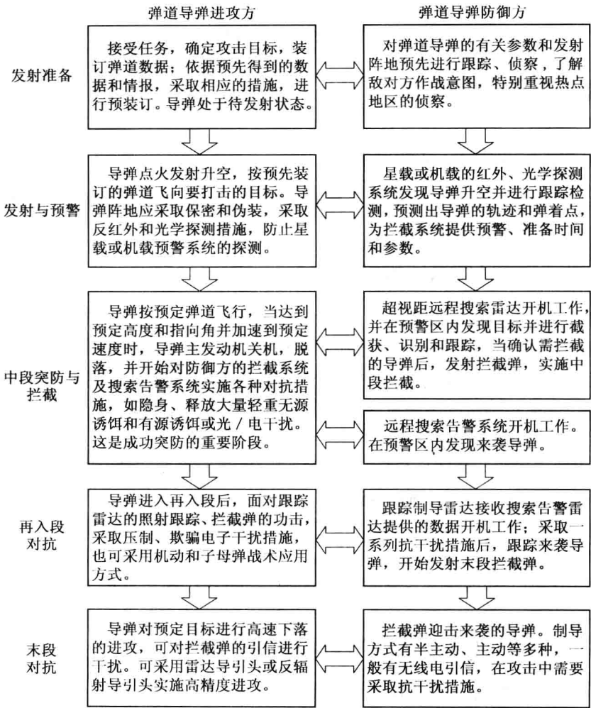
图 1-2 弹道导弹攻防对抗基本过程图
